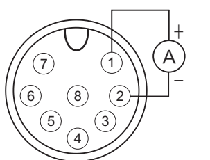
RS-485通訊協定電源配線圖
