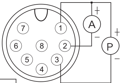
配線圖
