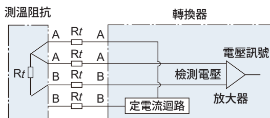
●P1-4線式溫度測量電路
